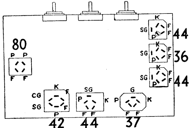
Fig. 1—Tube Sockets
